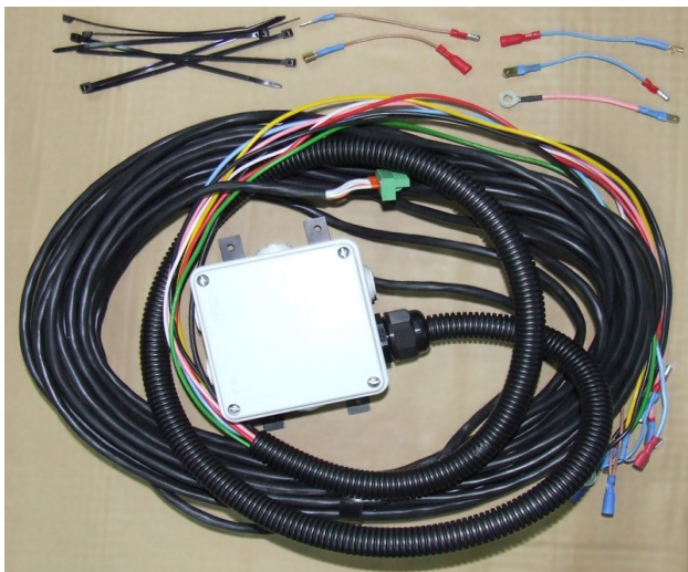
Рис.1. Блок электрики ИУ13с.
