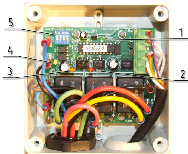
Рис.2. Блок ИУ13с (без верхней крышки).
