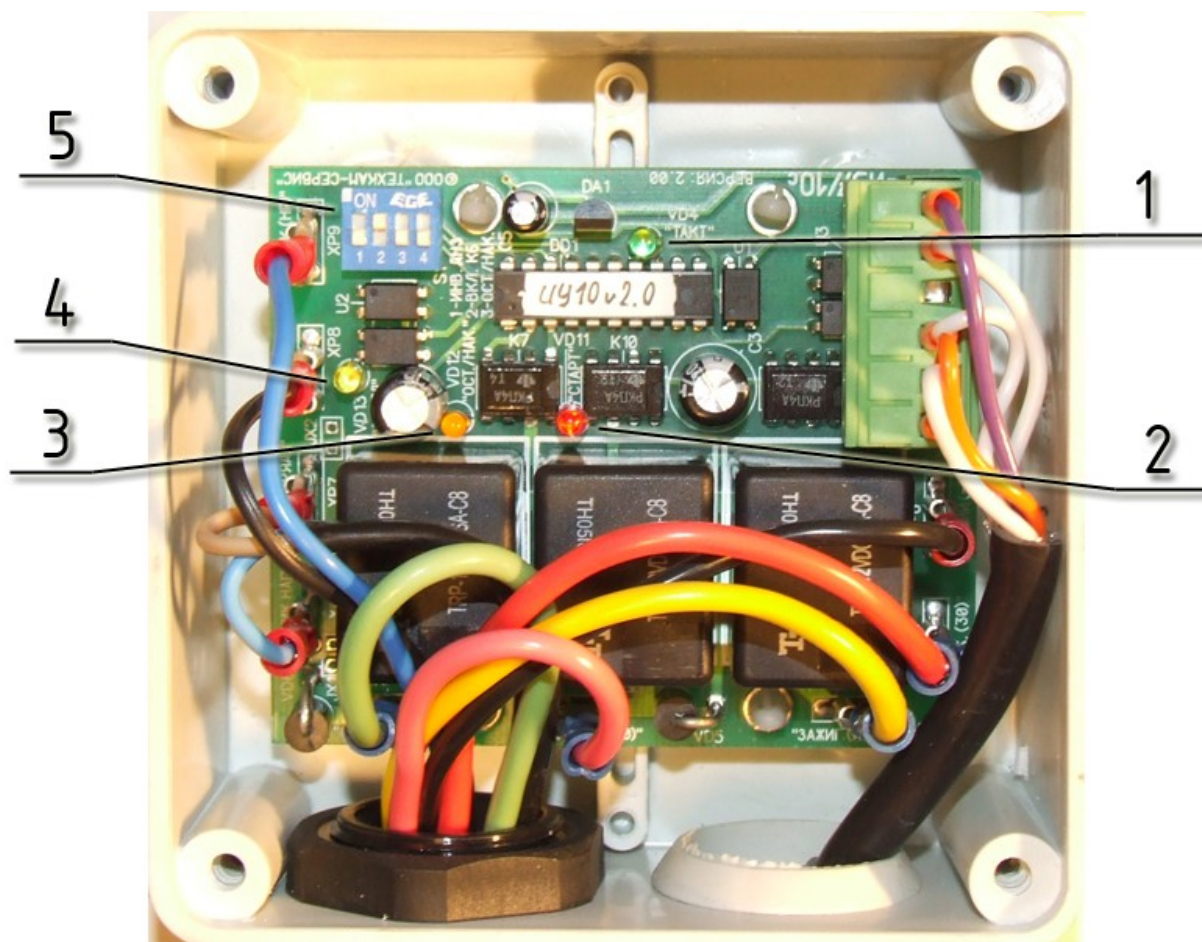
Рис. П2.1. Диагностика блока ИУ13с.
