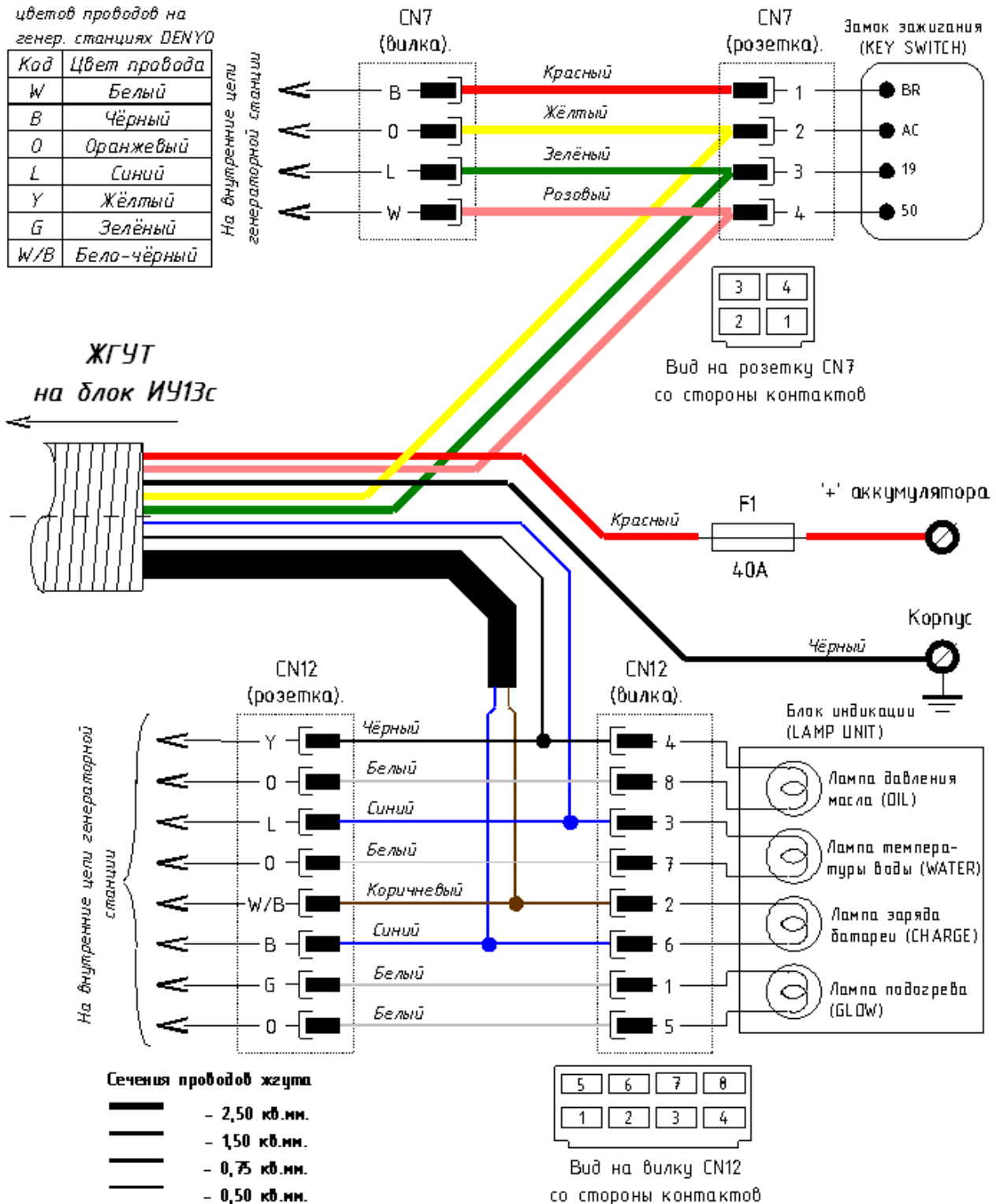
Рис. П1.2. Электрическая схема подключения комплекта ИУ13с к дизельным генераторным станциям TLG12ESX и TLG15ESX фирмы DENYO.
