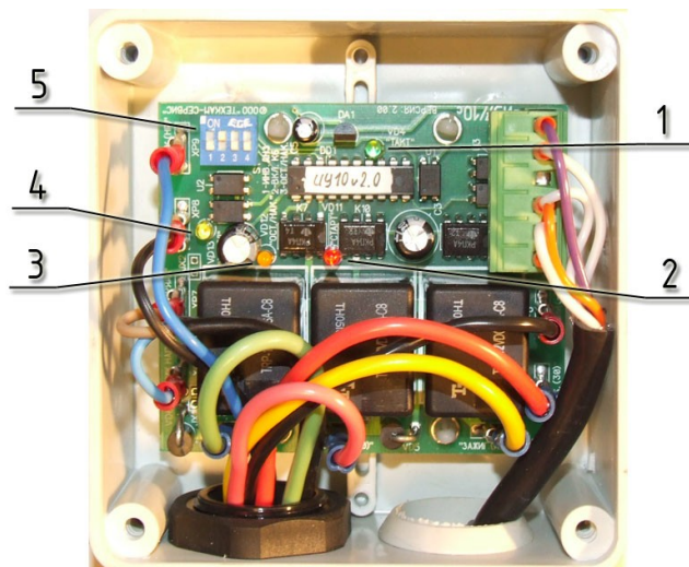
Рис.2. Блок ИУ14с (без верхней крышки).
