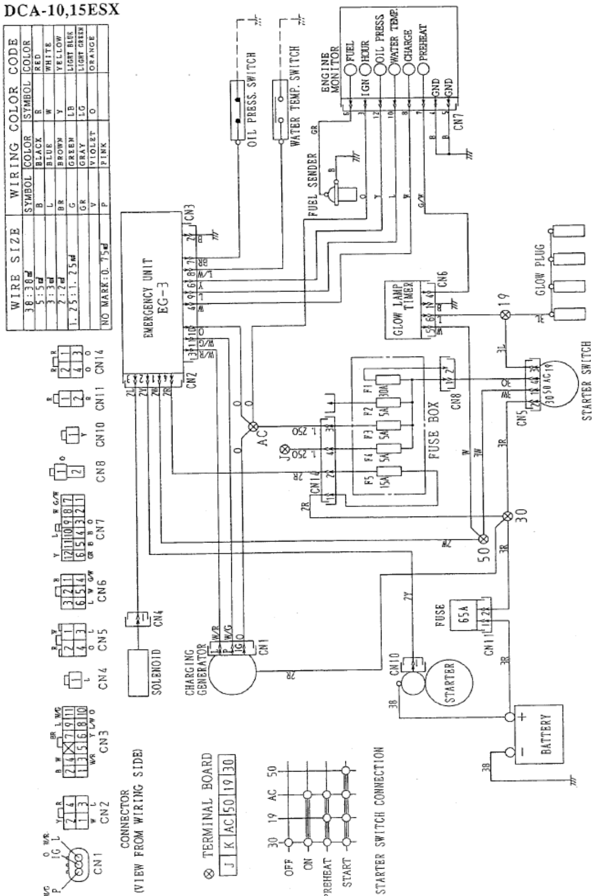
Рис.ПЗ.1. Схема электропроводки двигателей DENYO DCA-10ESX, DCA-15ESX.
