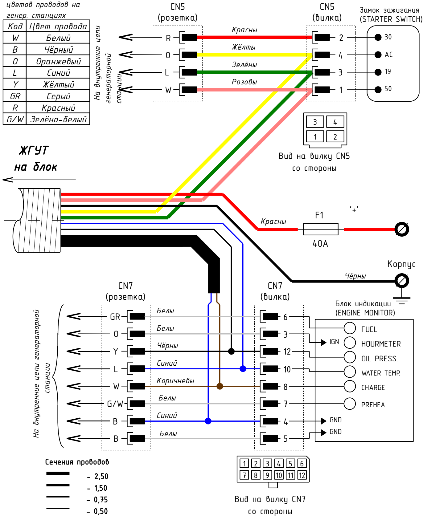
Рис. П1.2. Электрическая схема подключения комплекта ИУ14с к дизельным генераторным станциям серии DCA фирмы DENYO.
