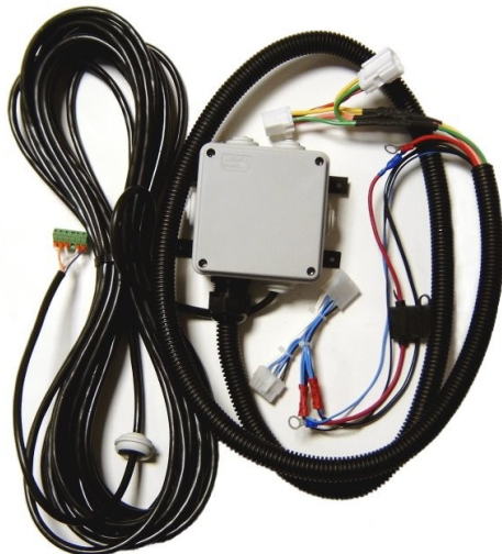
Рис.1. Блок электрики ИУ14с.
