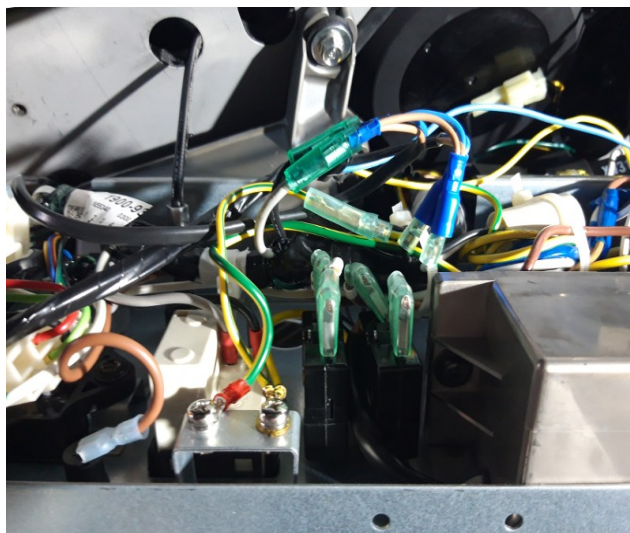
Рис. П2.15 Подключение провода питания привода к низковольтному фильтру генератора.
