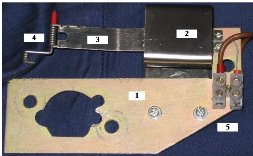
Рис.2. Электропривод воздушной заслонки.
