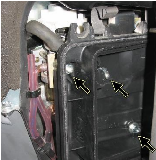
Рис. П2.1. Элементы крепления задней крышки воздушного фильтра.
