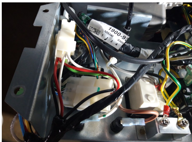
Рис. П2.14. Подключение разъемов жгута к проводке и размещение внутри панели ГС.
