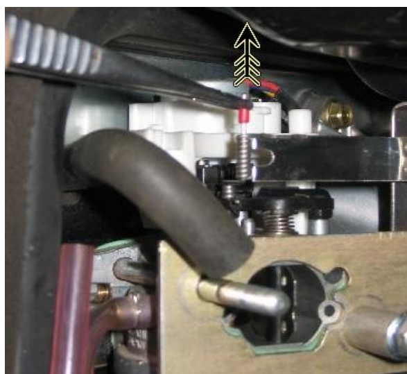
Рис. П2.7. Поднятие тяги привода.
