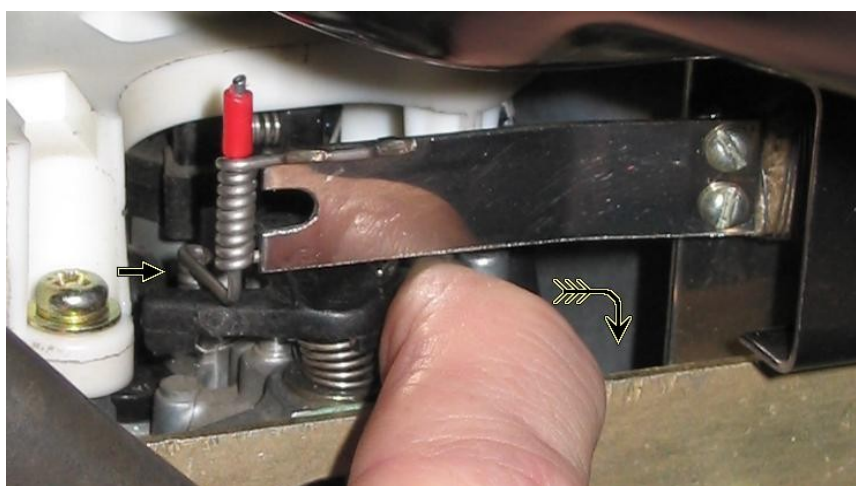
Рис. П2.9. Возврат заслонки с тягой.
