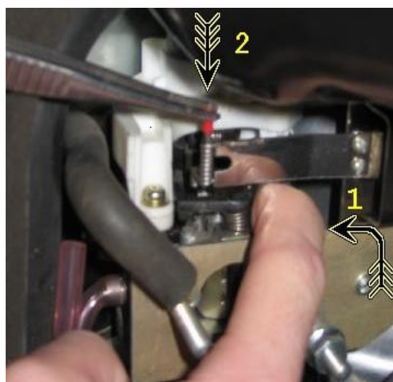
Рис. П2.8. Поворот заслонки и зацепление.
