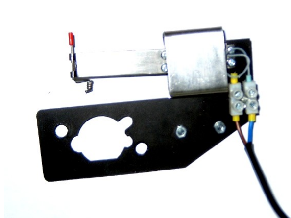
Рис. П2.6. Подключение проводов питания.
