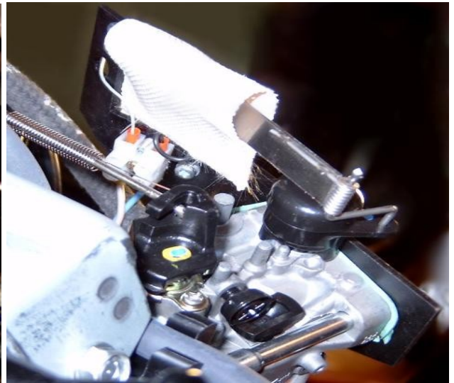
Рис.5, Рис.6. Вид на установленный электропривод GX240-GX390.
