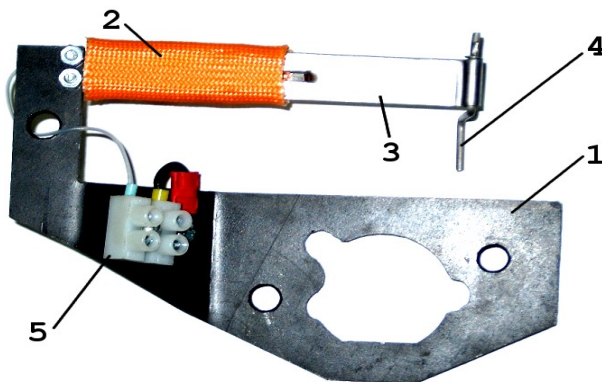
Рис.1. Электропривод воздушной заслонки ПБЗ-10 (слева) для двигателей GX240-GX390 с полуавтоматической заслонкой (с вакуумным клапаном) (внешний вид двигателя справа).
