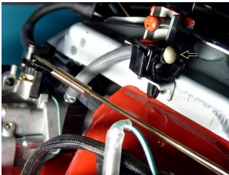
Рис.7. Установка заглушки.
