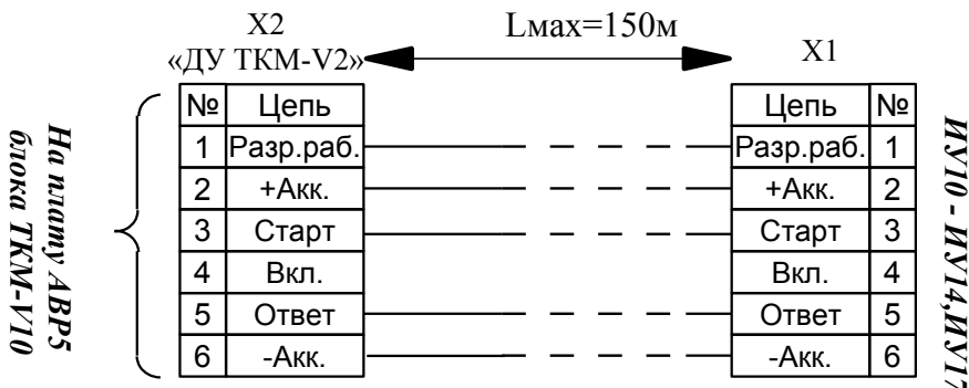
Схема №1. Подключение исполнительных устройств из серии ИУ10 — ИУ14, ИУ17.
