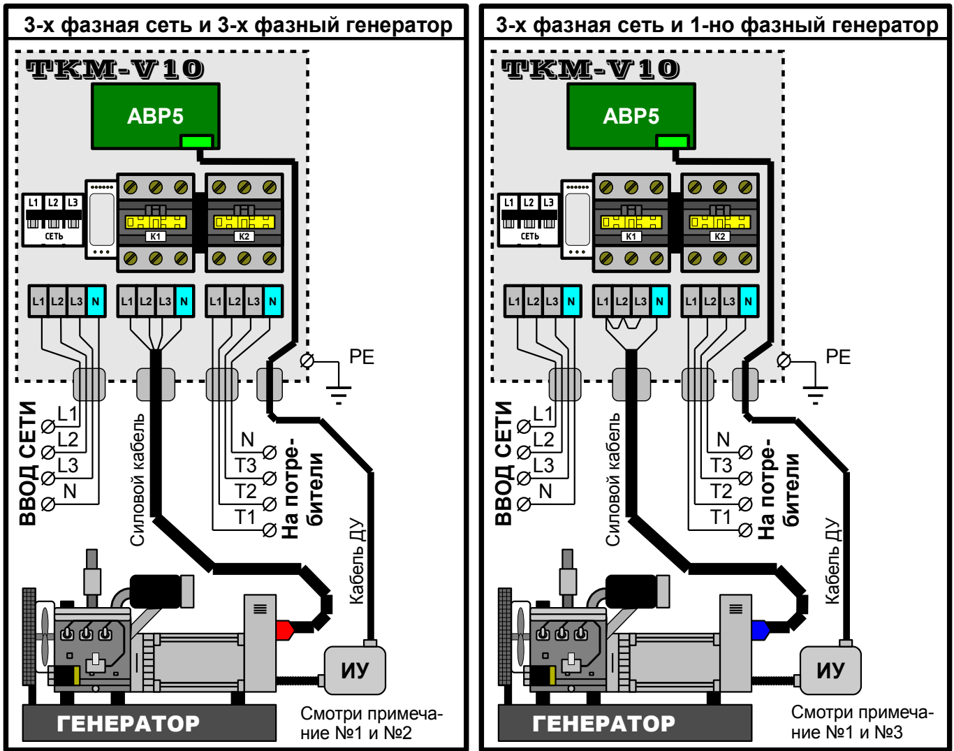
Рис.4. Варианты подключения силовых цепей блока ТКМ-V10.
