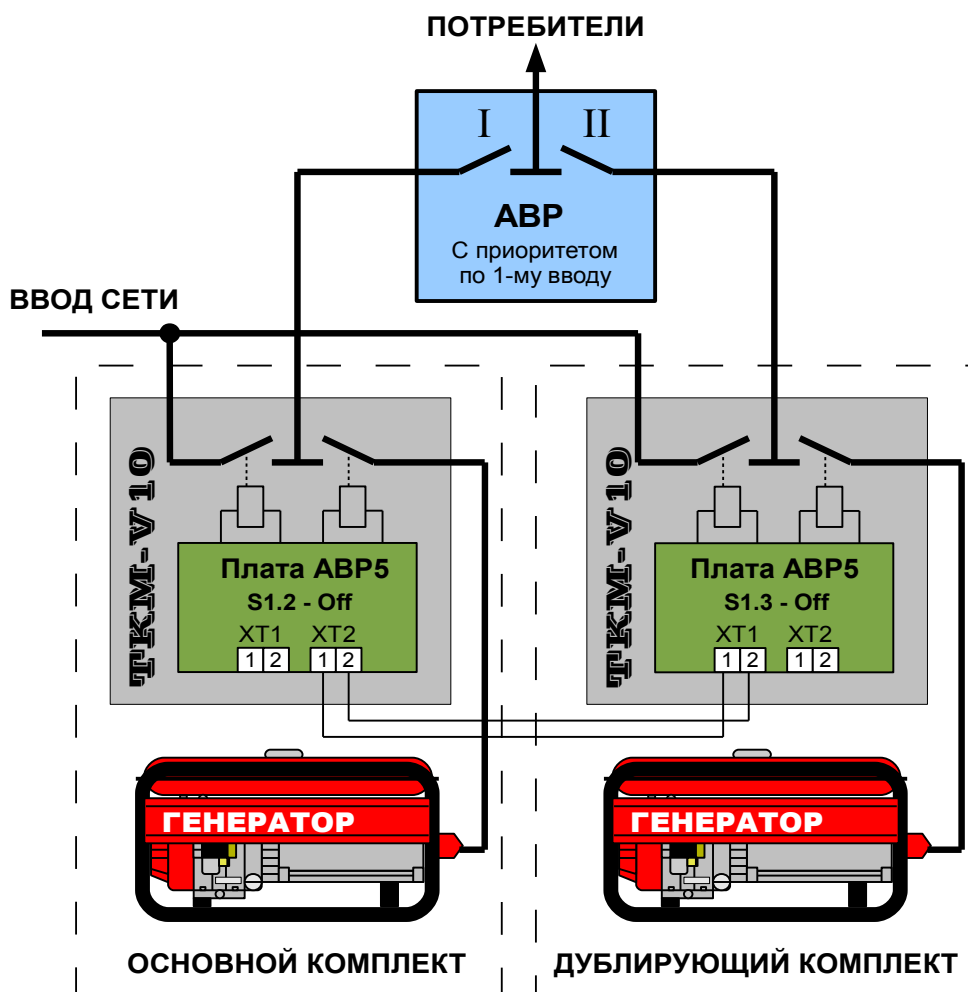
Рис.5. Пример системы с дублированием резервного электроснабжения.
