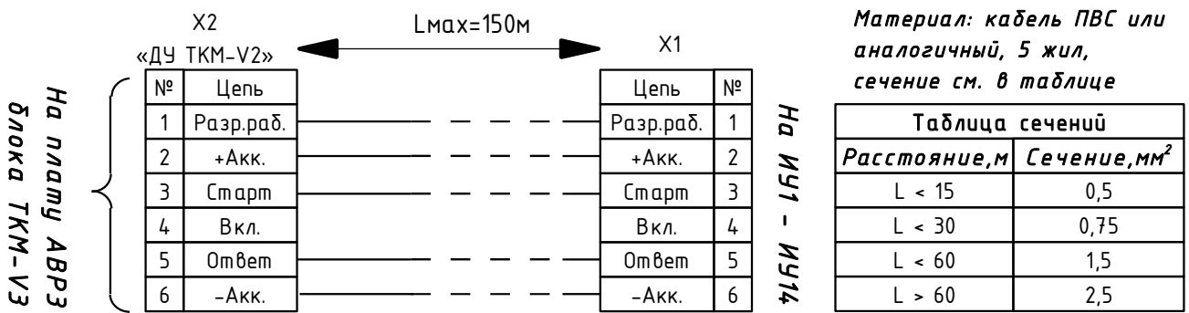
Схема №1. Подключение исполнительных устройств из серии ИУ1 – ИУ14.
