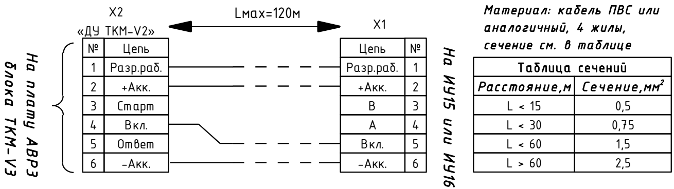
Схема №2. Четырёх-проводная (при ЗУ расположенным в шкафу коммутации ТКМ).
