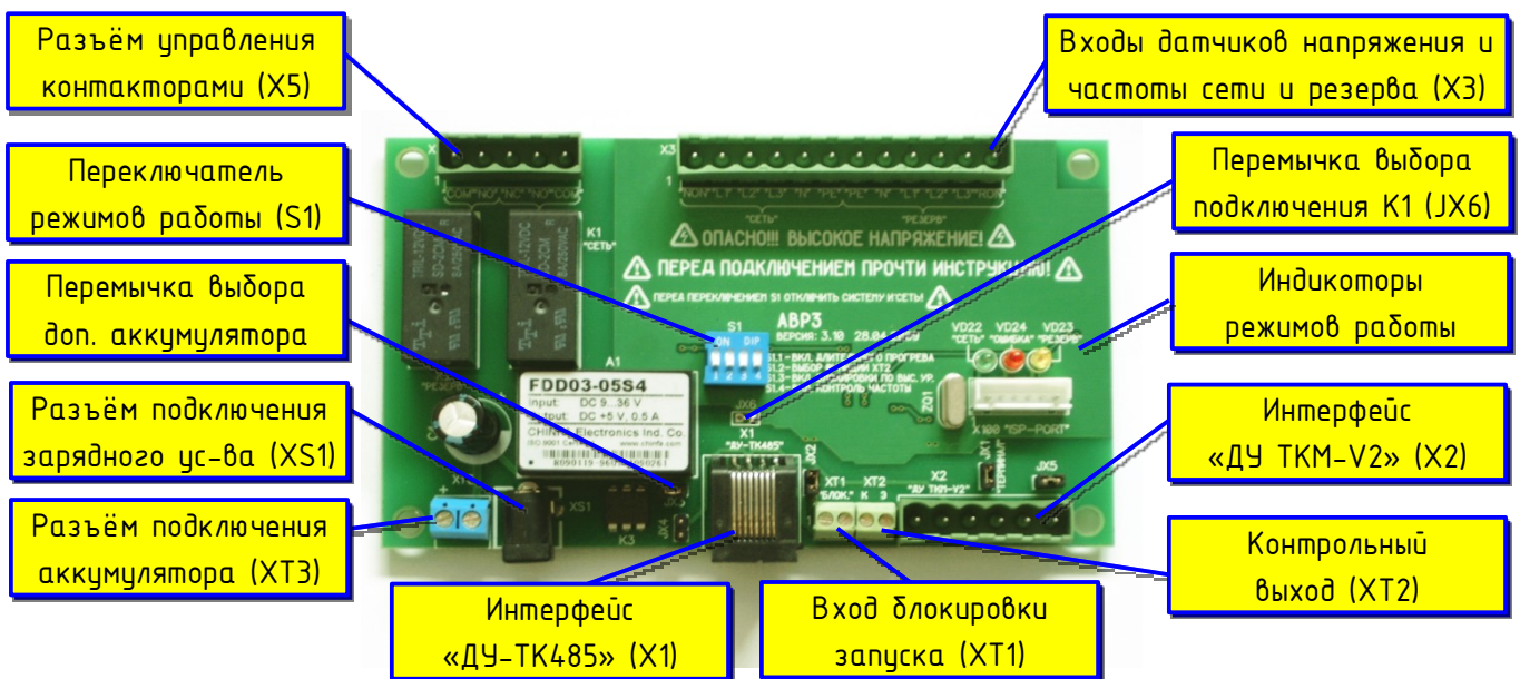
Рис.П2.1. Внешний вид платы АВР3.
