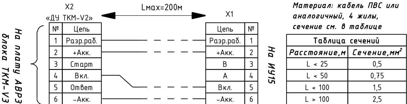
Схема №3. Четырёх-проводная (при ЗУ расположенном в ИУ15с).
