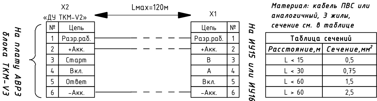
Схема №4. Трёхпроводная с отдельным включением ИУ и ТКМ (ЗУ расположено в шкафу коммутации ТКМ).
