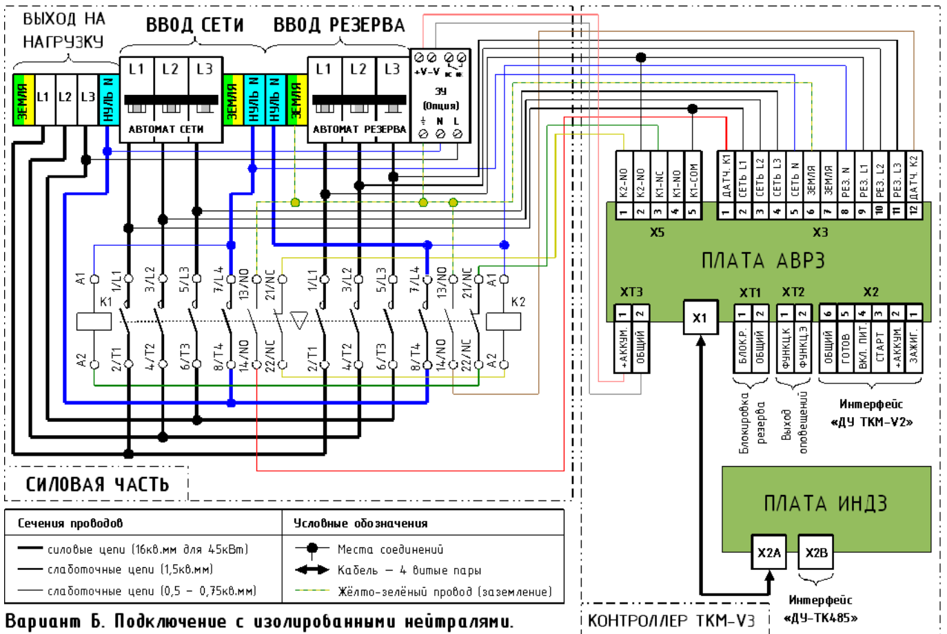
Рис.3. Варианты разводки шкафа коммутации и подключения к нему контроллера ТКМ-В3.
