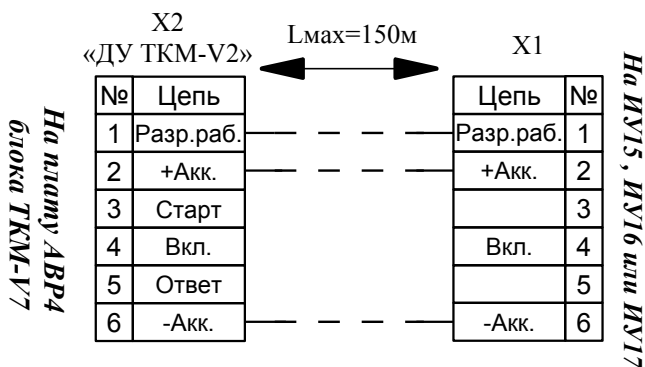
Рис.8. Подключение исполнительных устройств ИУ15, ИУ16 и ИУ17.
