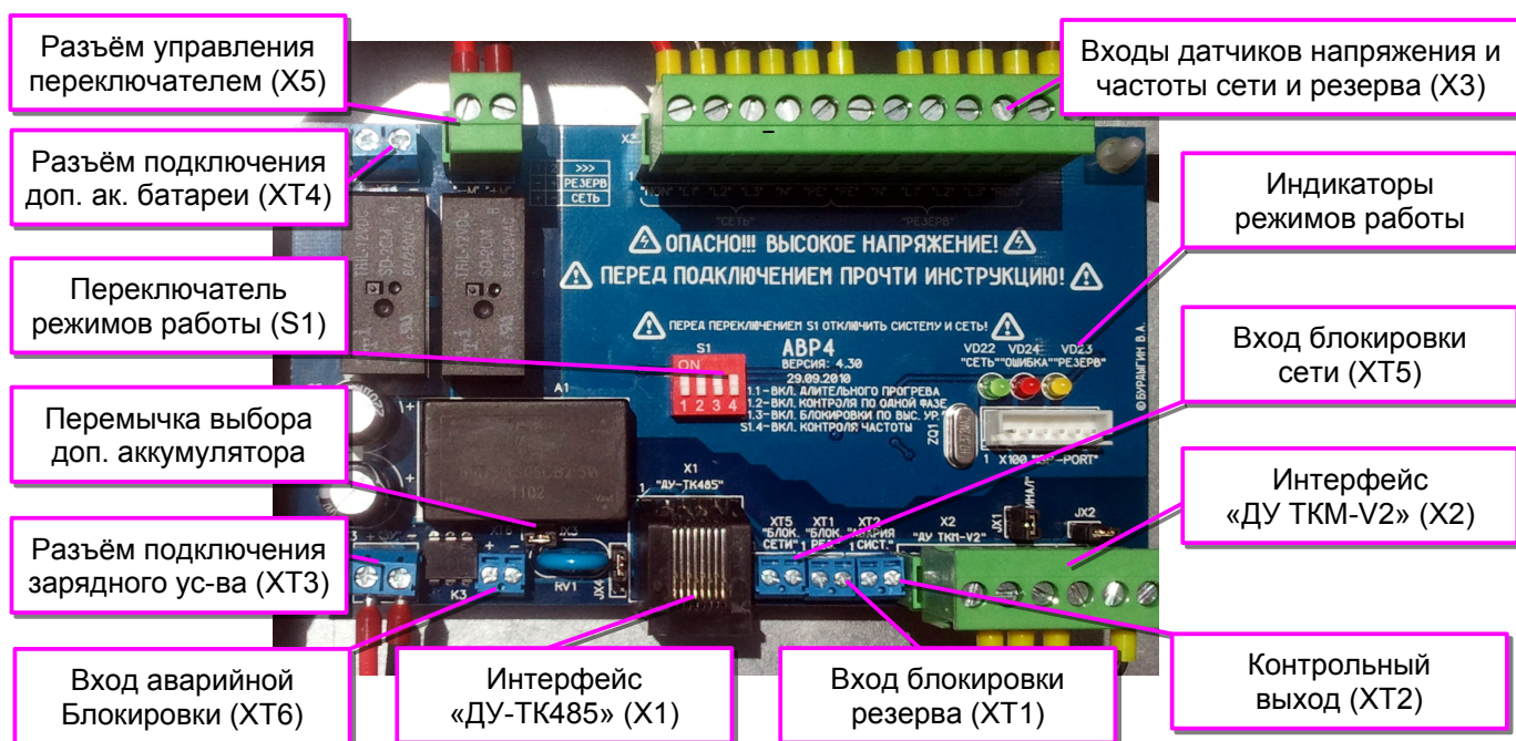
Рис.П2.1. Внешний вид платы АВР4.
