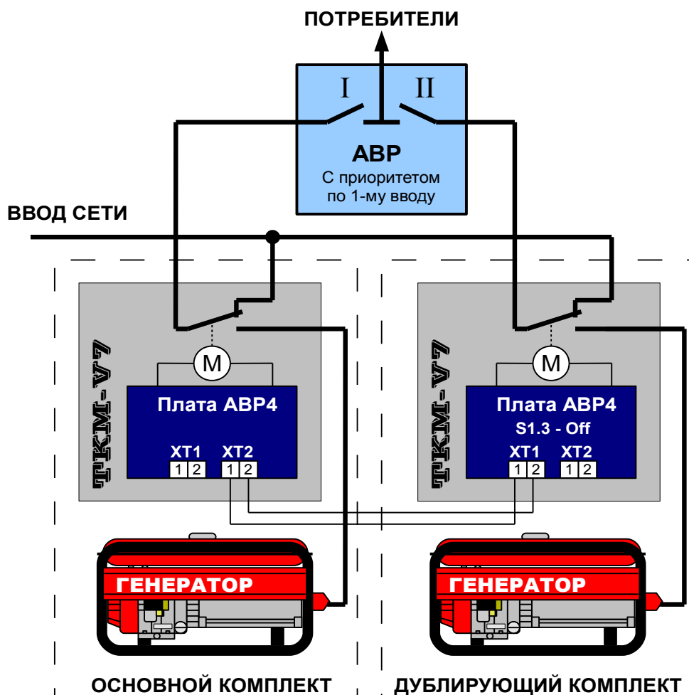
Рис.9. Пример системы с дублированием резервного электроснабжения.
