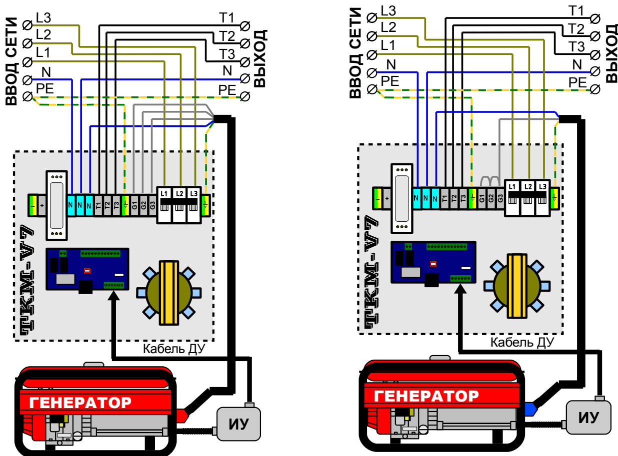
Рис.3. Схема шкафа ТКМ-V7.
