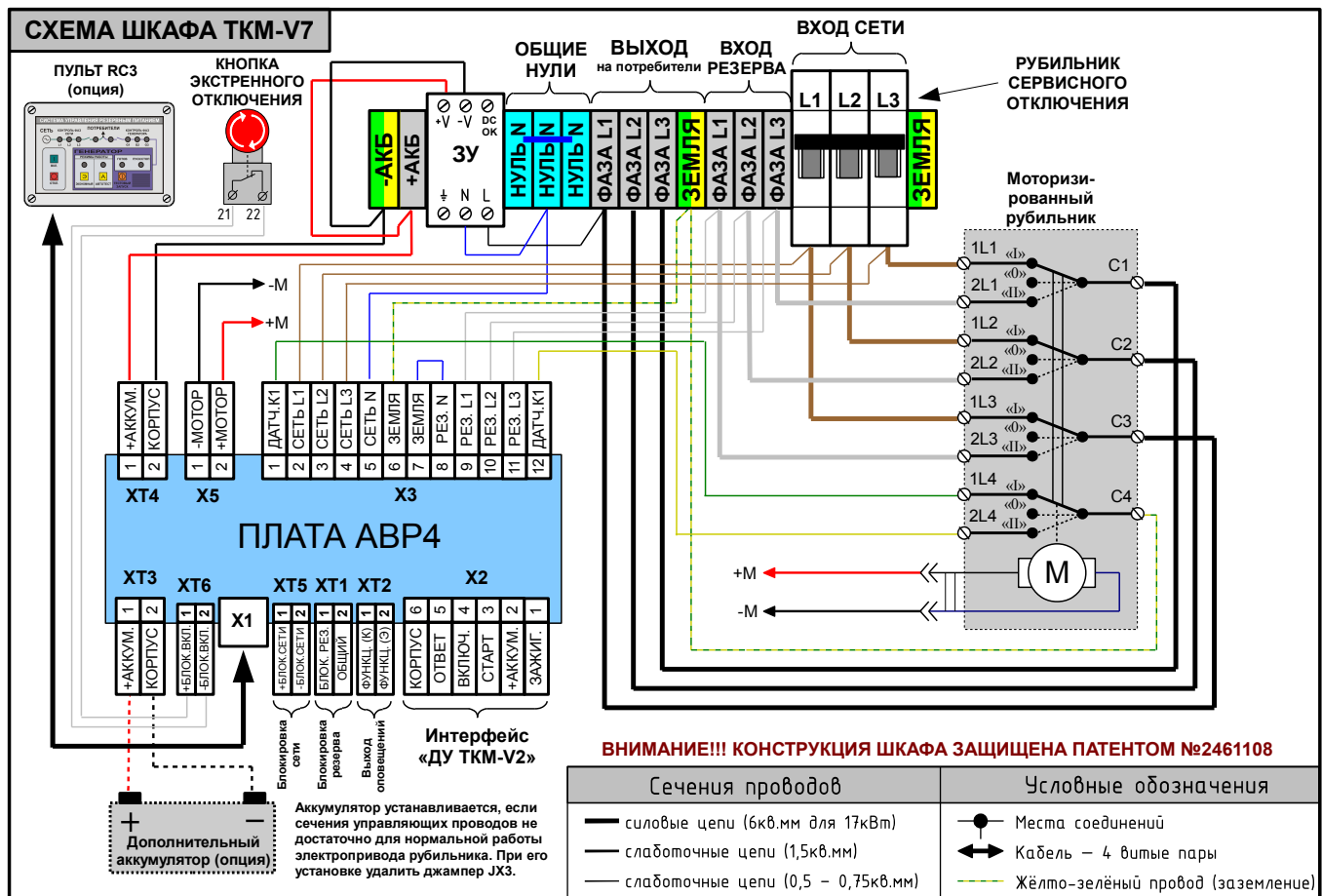
Рис.3. Схема шкафа ТКМ-V7.
