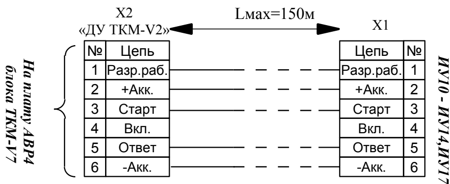
Рис.7. Подключение исполнительных устройств из серии ИУ1 — ИУ14, ИУ17.
